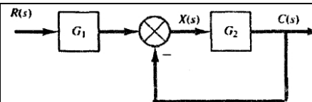
图 1 系统结构图
