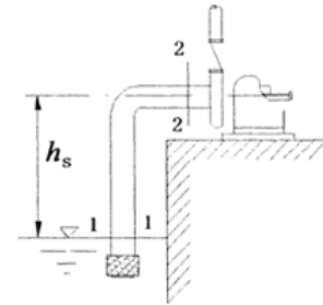
图 6-11 水泵吸水管
