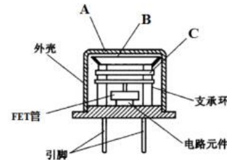
图 3 热释电红外传感器结构图
