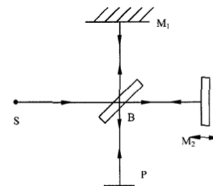
迈克尔逊干涉系统原理图
