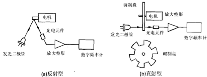
光电转速传感器工作原理图
