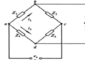
图 4 交流电桥电路
