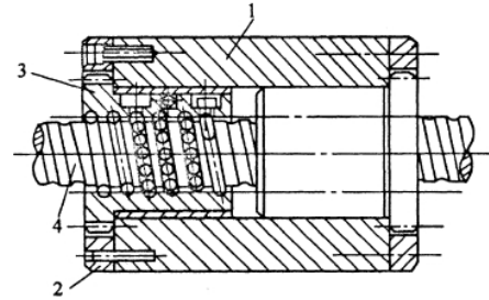
1—套筒 2—内齿轮 3—圆柱齿轮 4—丝杠
