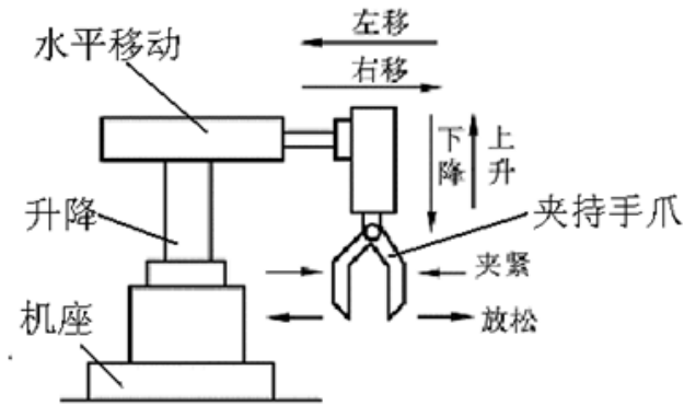
物料搬运机械手结构原理图
