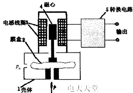
图 气体压力传感器
