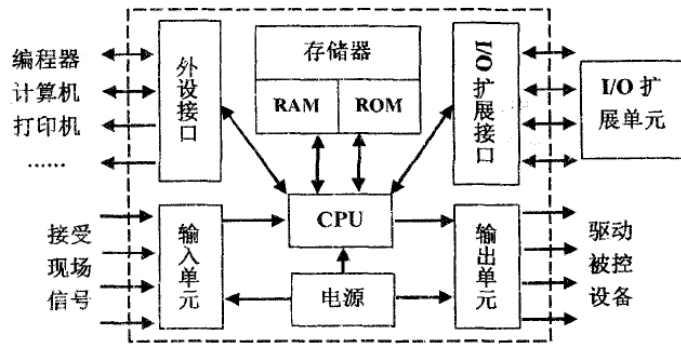
图 PLC 的组成结构框图
