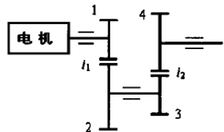
图电动机驱动的二级齿轮传动减速传动系统
