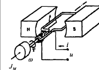
图直流电动机的工作原理
