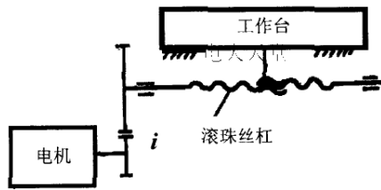
图电机驱动工作台示意图
