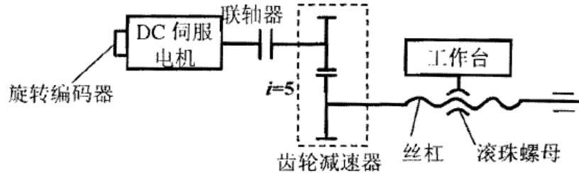
图直流电机丝杠螺母机构驱动工作台
