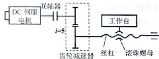
图直流电机丝杠螺母机构驱动工作台示意图
