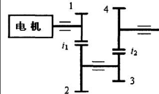
图电动机驱动的二级齿轮传动减速传动系统图
