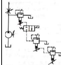
图 1 远程三级调压液压回路
